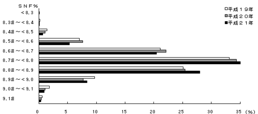
図6 SNFの分布
